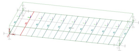
Verteilung mit individuell gewählten Einflussbreiten
