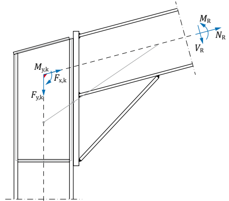
Lastvektoren der Rahmenecke
