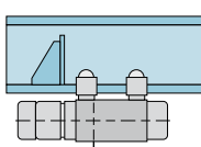
Katzbahnträger
