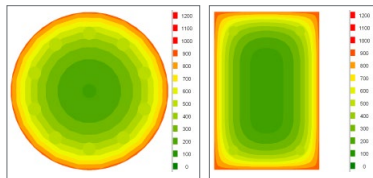
Beispiel: R120 für runde und rechteckige Querschnitte
