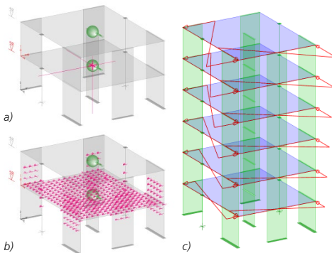
a) Ersatzlasten in selektierten Auswertungsraum
