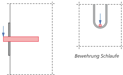
Scherbolzen mit angeschweißter Stahlplatte
