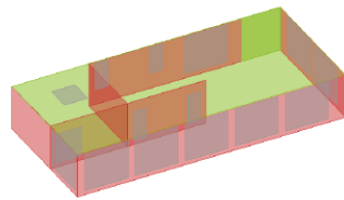
Berechnungsmodell für Staffelgeschoss
