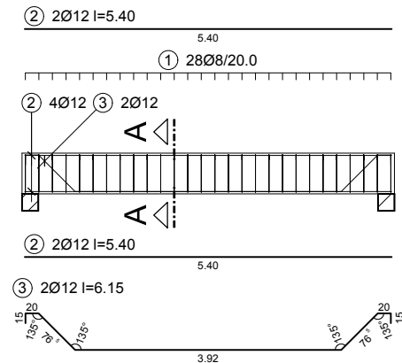
Feldbewehrung mit Schubaufbiegung
