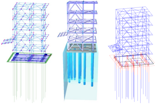
Gesamtsystem mit Pfahlgründung
