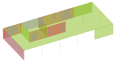
Berechnungsmodell für Decke über 3. OG
