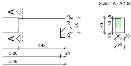
Schalplanausschnitt: Träger mit Querschnittsprung und Versatz
