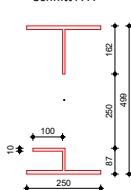
Schnitt A-A
