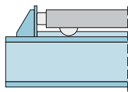
Kranbahnträger
