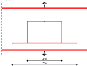
Stahl-Trägeröffnung Ansicht
