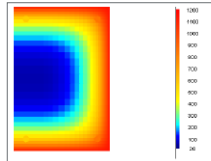
Für Rechteckquerschnitte sind alle Beflammungssituationen – auch dreiseitig (Beispiel) oder über Eck – möglich.
