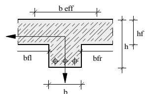
b) Unterzug
