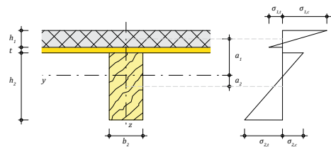
Spannungsverteilung im Verbundquerschnitt
