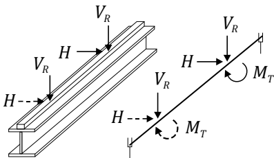
Prinzipielle Belastung eines Kranbahnträgers
