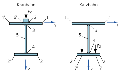
Nachweispunkte des Trägerquerschnitts
