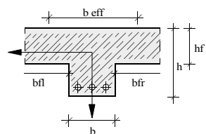
b) Unterzug
