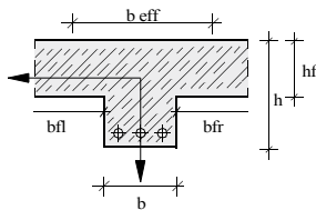
b) Unterzug
