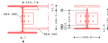
Anschluss mit Winkeln
