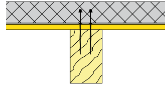
Verbundquerschnitt
