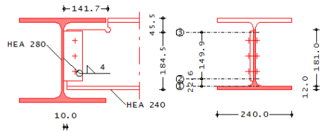
Anschluss mit Fahnenblech
