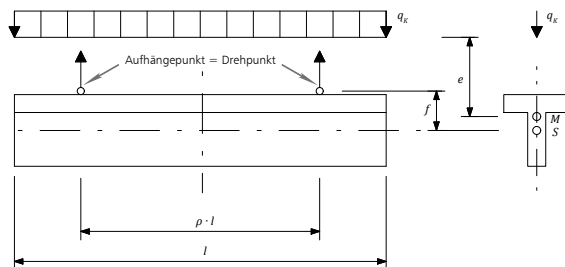
Berechnungsmodell für den kippgefähr- deten, aufgehängten Träger nach Lebelte [(Lebelte); Deneke, O., Holz, K. und Litzner, H.-U.: Übersicht über praktische Verfahren zum Nachweis der Kippsicherheit schlanker Stahlbeton- und Spannbetonträger. Beton-Stahlbetonbau. Ausgabe Heft 9, 1985.]
