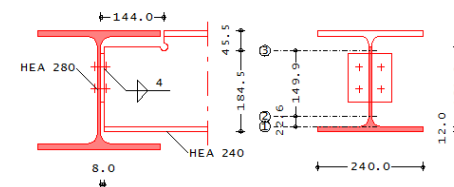
Anschluss mit Stirnplatte
