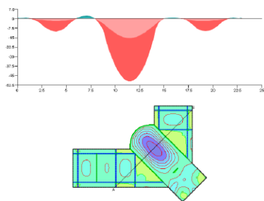
Vergleich Endverformung f_{\infty} im Zustand I und Zustand II
