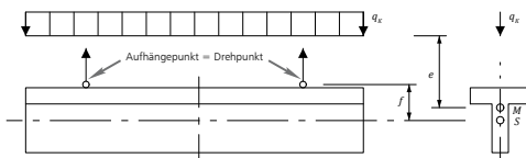
Berechnungsmodell für den kippgefährdeten, aufgehängten Träger nach Labelle
